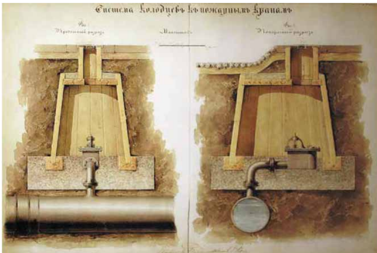
Схема водопровода, XIX в.
