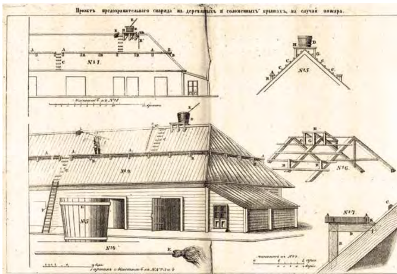
Проект предохранительного снаряда на деревянных и соломенных крышах на случай пожара. 1849 г. 7
