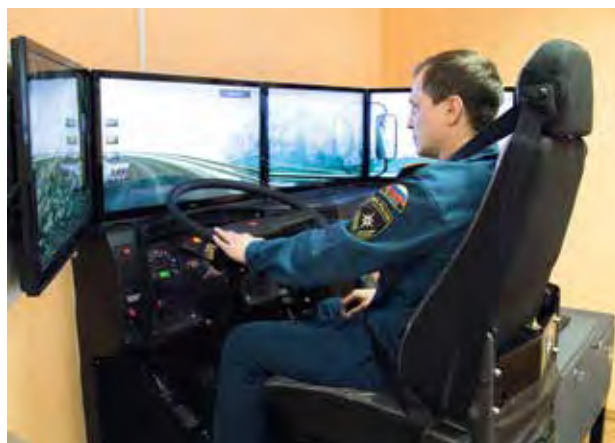
Тренажер отработки элементов управления пожарной машиной в особых условиях «КАМАЗ—МАСТЕР МЧС ОЗ\АР»
